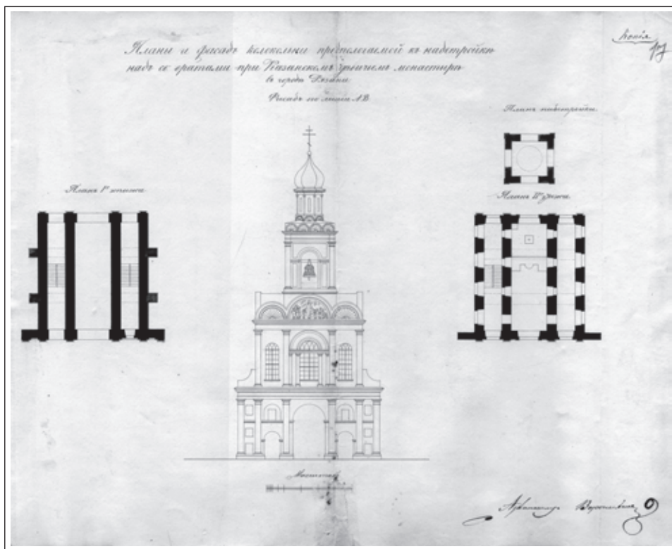
План и фасад монастырской колокольни с Варварьинским храмом и Святыми воротами. 1870-1872 годы. Автор — Рязанский губернский архитектор Николай Ильич Воронихин. Из фондов ГАРО
